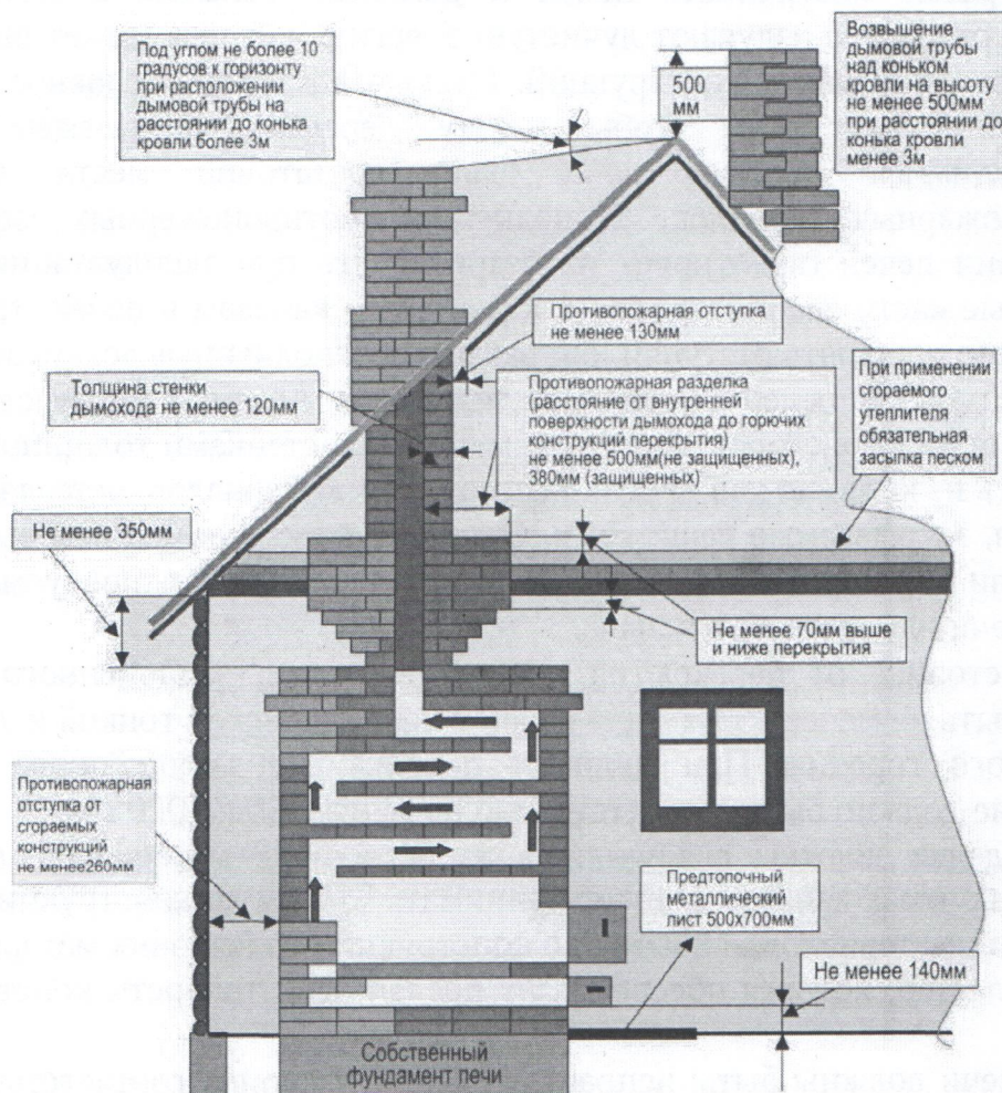
Рисунок 1. Схема безопасного устройства печи.
